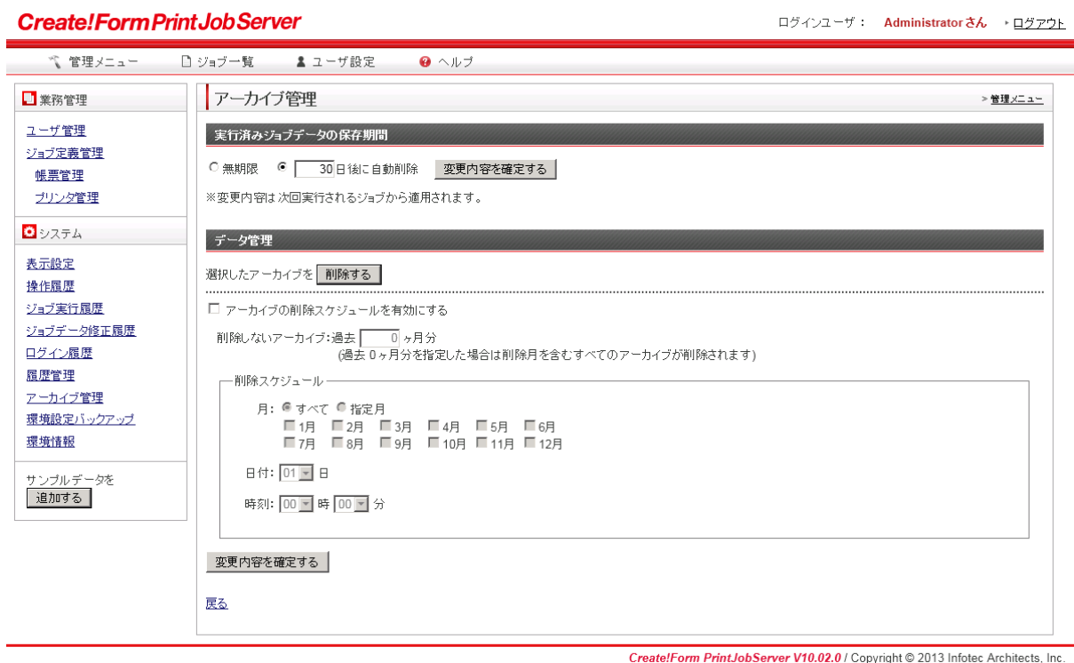
図 3.5 アーカイブ管理画面
